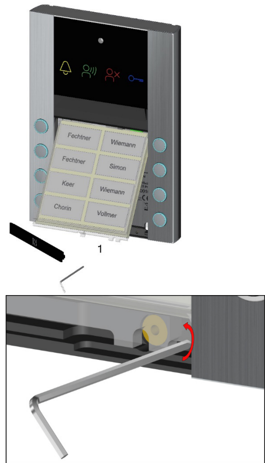
Abb. 8: Namensschildmodul entfernen
