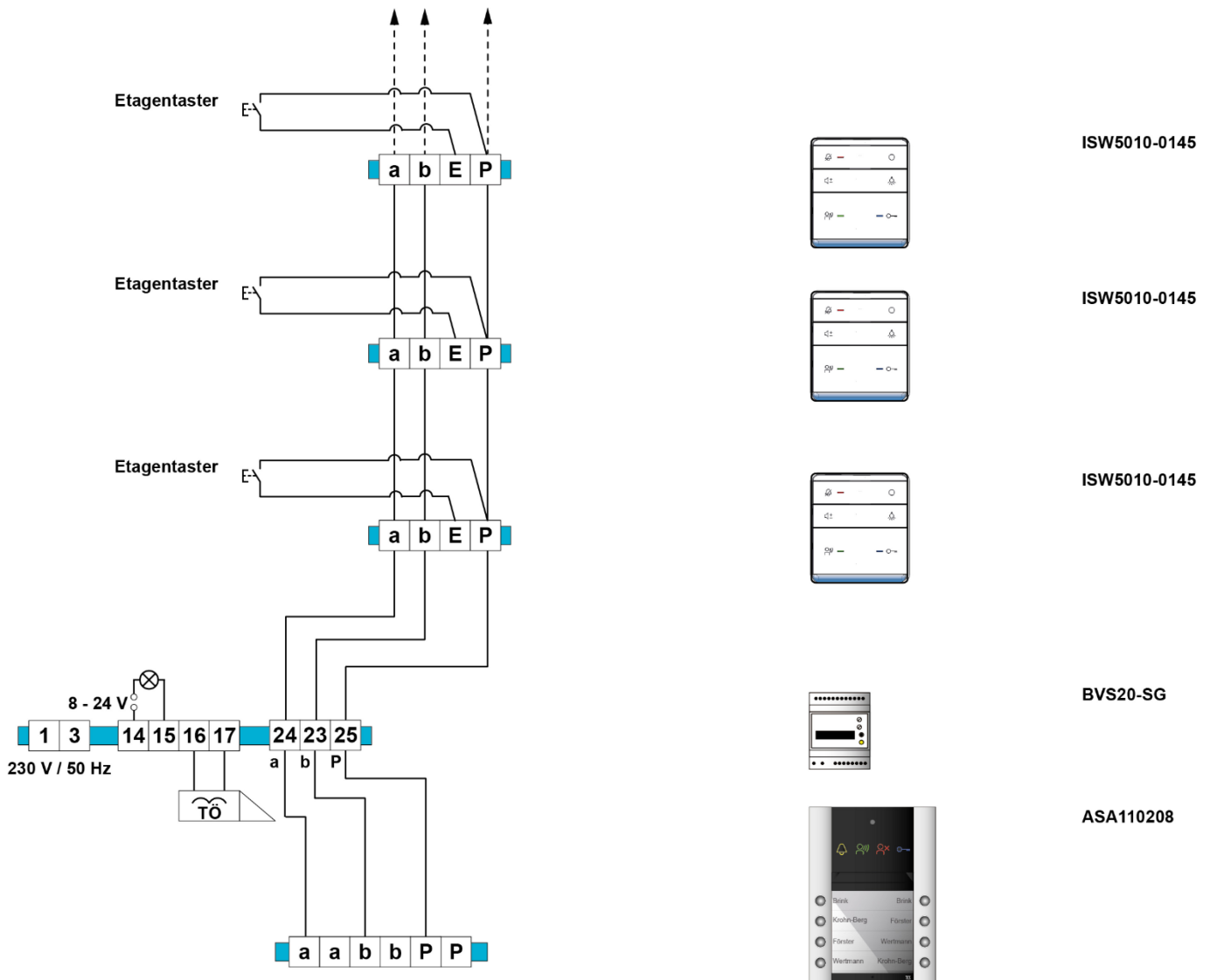
Abb. 14: Schaltungsbeispiel für Audio-Außenstation ASA1...
