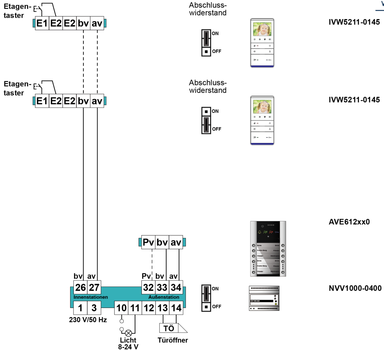
Abb. 16: Schaltungsbeispiel für Video-Außenstation AVA6... Video-2-Draht:BUS
