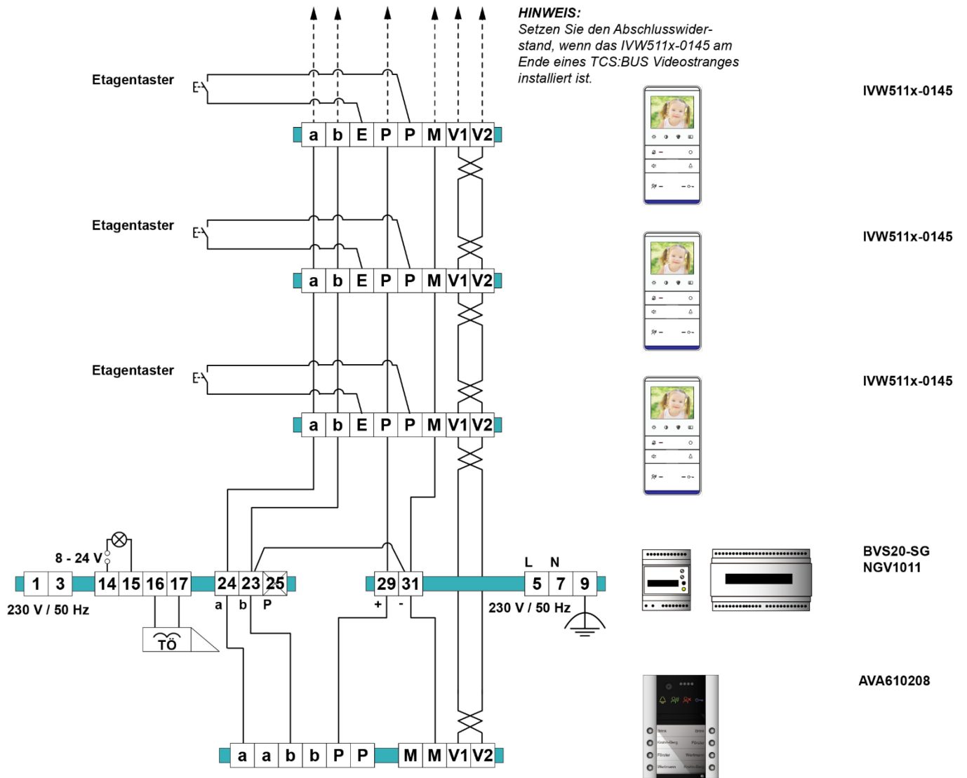
Abb. 15: Schaltungsbeispiel für Video-Außenstation AVA1...
