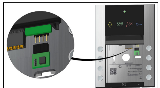
Abb. 20: Backup-EEPROM entfernen
