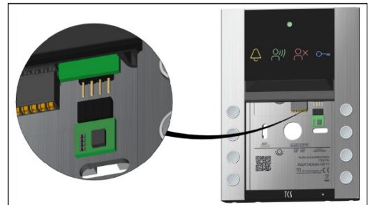
Abb. 18: Backup-EEPROM entfernen
