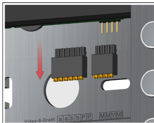
Abb. 11: Anschlussklemme abziehen
