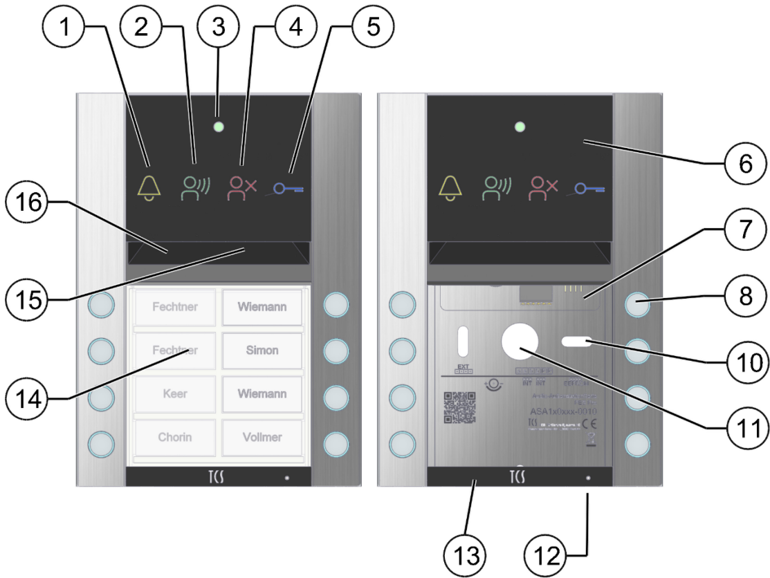
Abb. 1: Geräteübersicht
