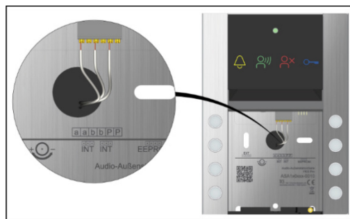
Abb. 12: Anschluss ASA
