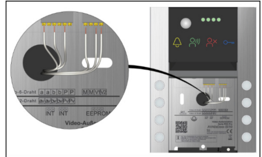
Abb. 13: Anschluss AVA
